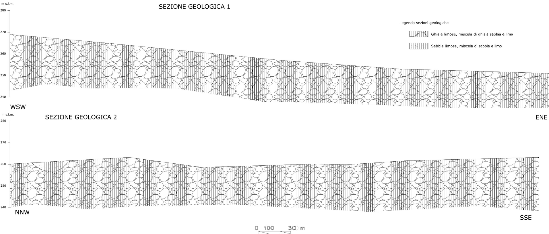
SEZIONE GEOLOGICA 1
